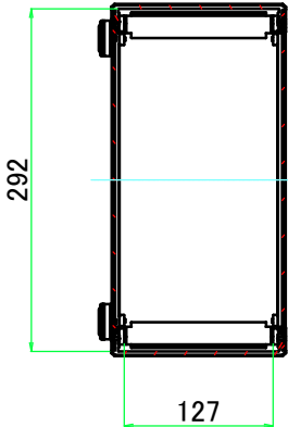
B-B ( 1 : 7 )
