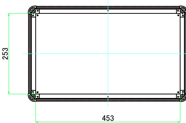
C-C ( 1 : 7 )
